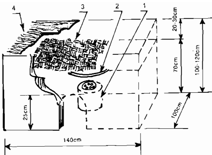
Hình 9. Cấu tạo lò sấy vải
